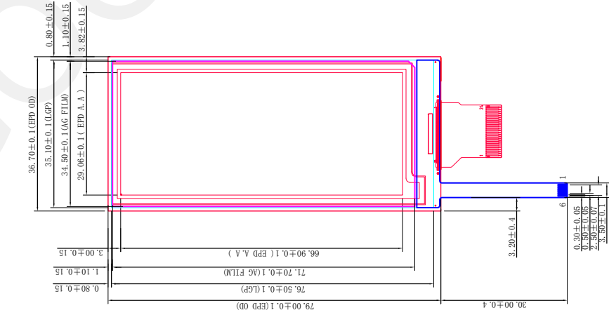
前视图 1:1
